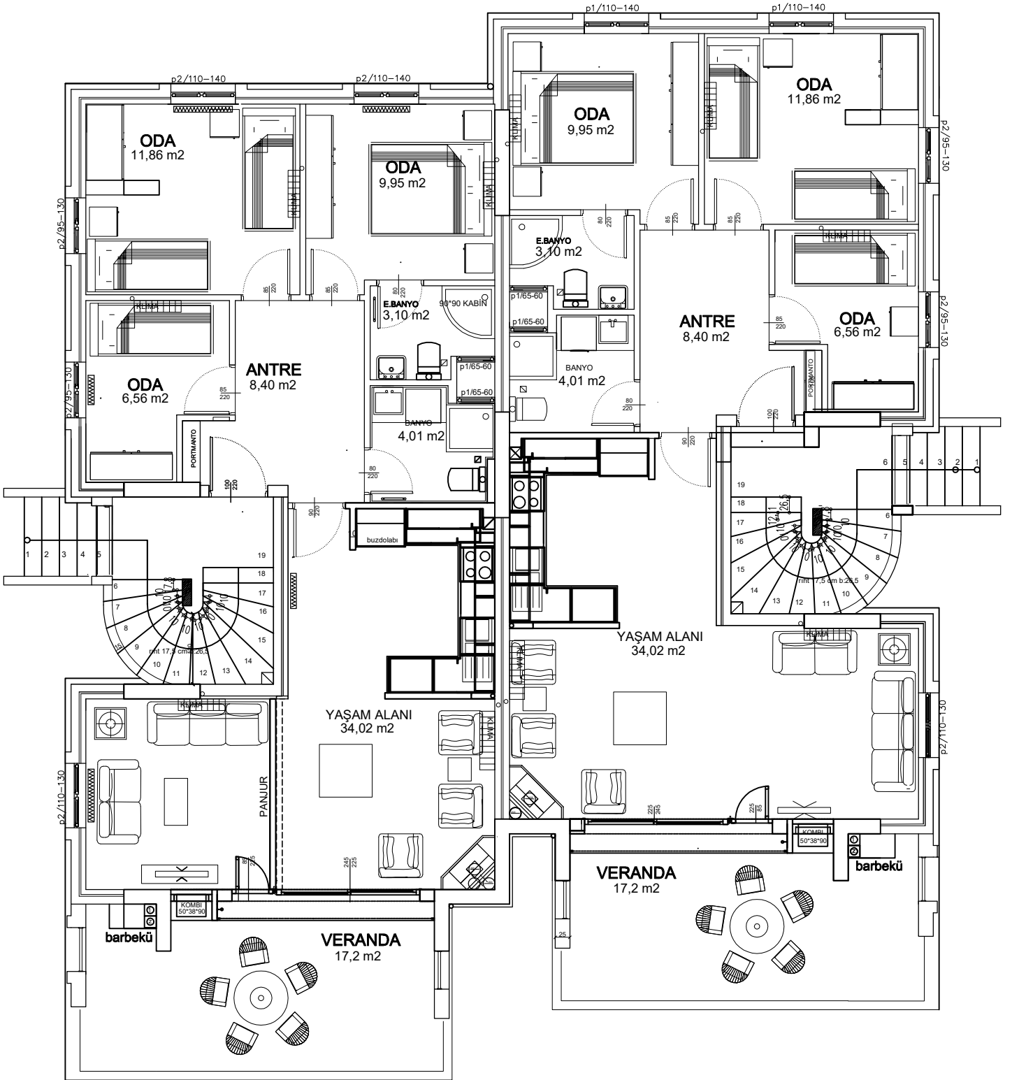
BİRİNCİ KAT PLANI
