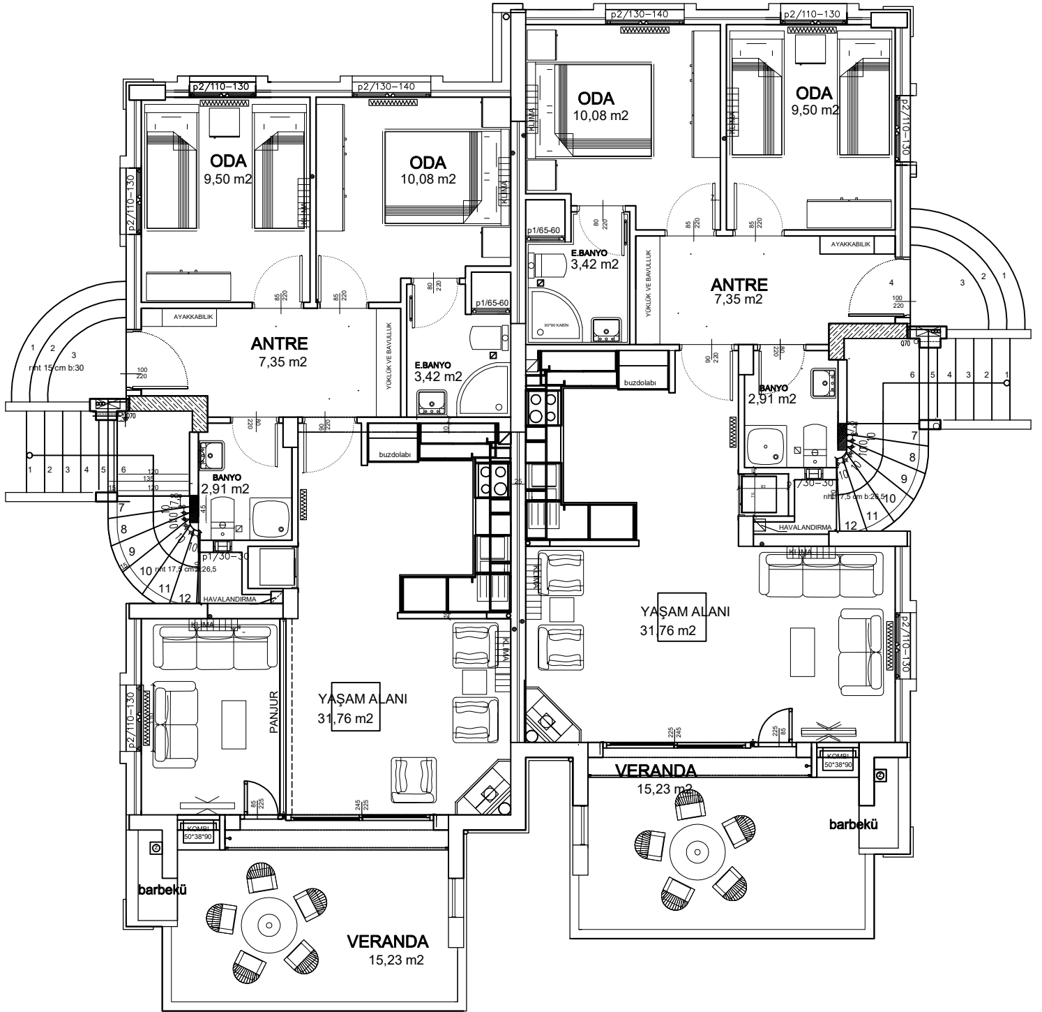
ZEMİN KAT PLANI
